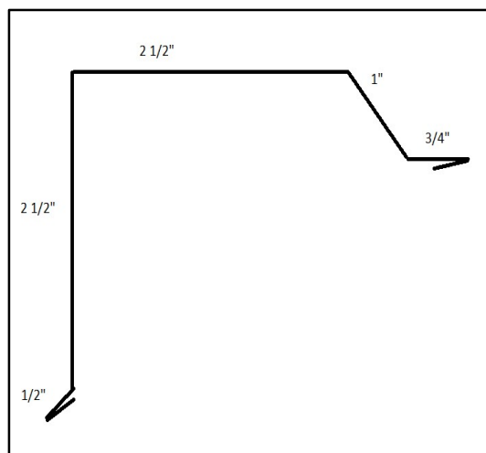
BARN RAKE
