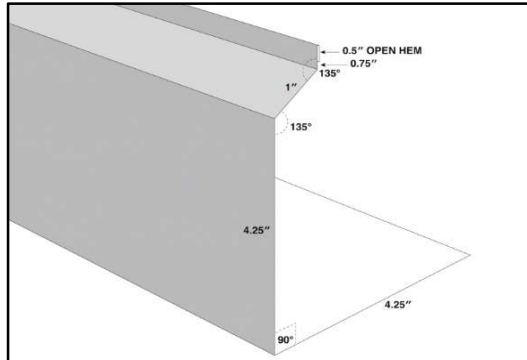
DOOR EDGE
