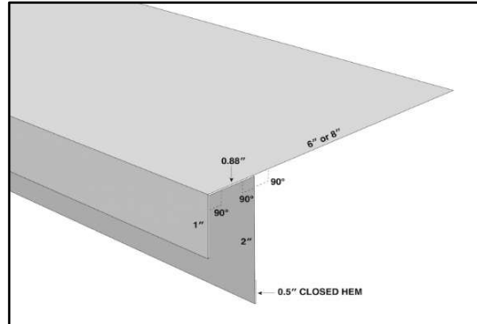
OVERHEAD DOOR JAMB
