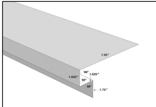
DOOR JAMB WIDE
