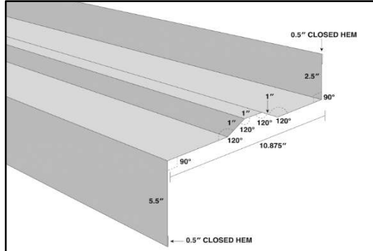
SOFFIT
