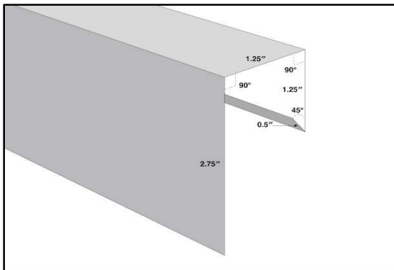
JAMB TRIM
