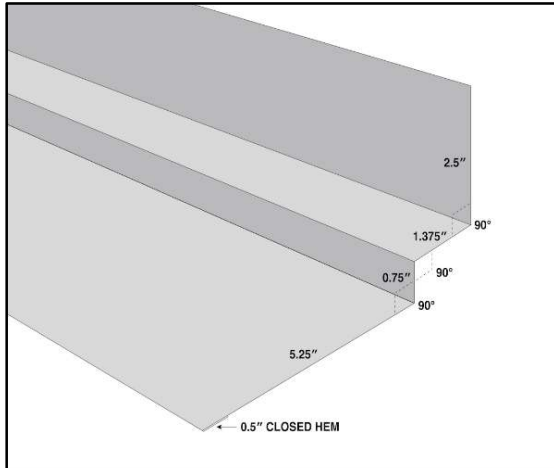
TIE-IN
