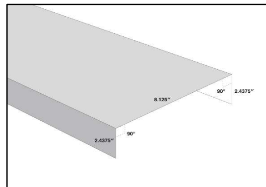
JAMB HEADER
