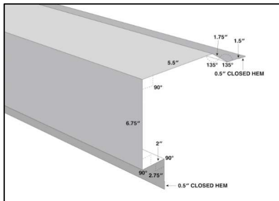
BOX RAKE
