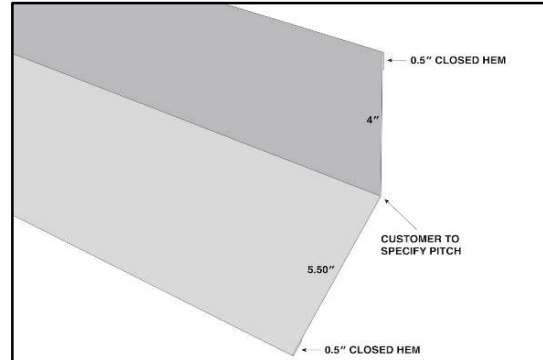
HI-SIDE PARAPET
