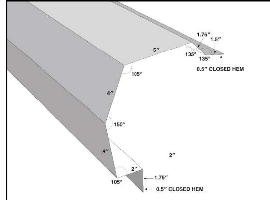
RAKE
